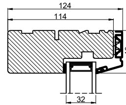
Lodret snit A
